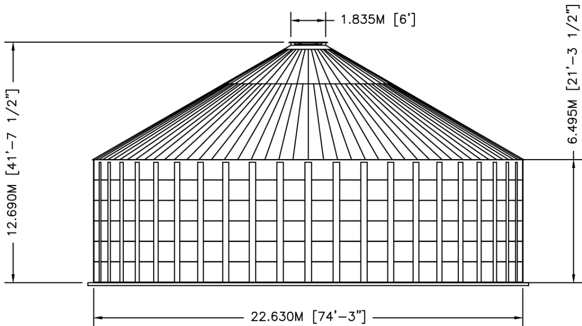
ELEVATION
